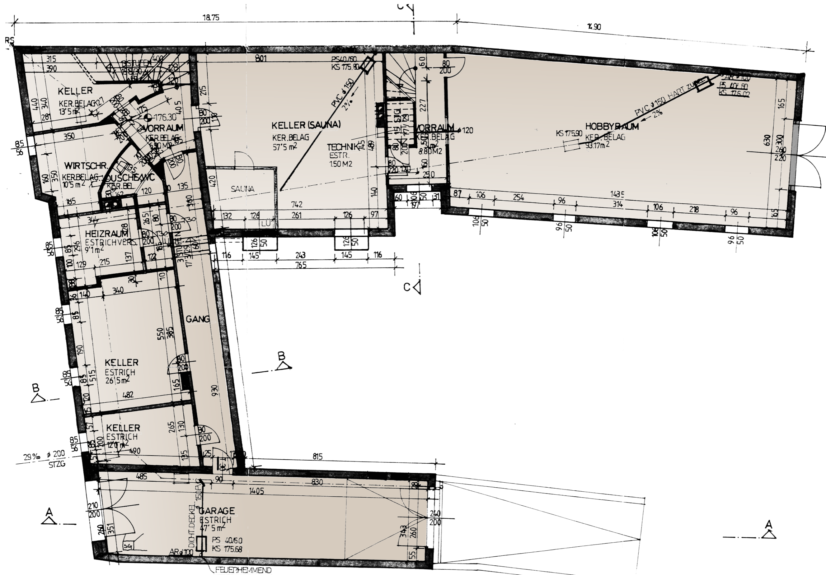
GRUNDRISS KELLERGESCHOSS
