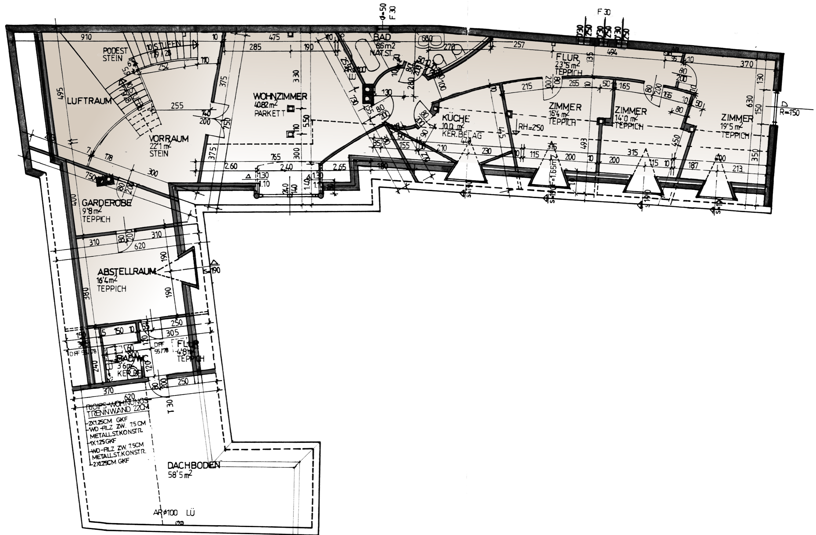
GRUNDRISS DACHGESCHOSS
